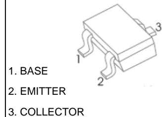
SOT-323
