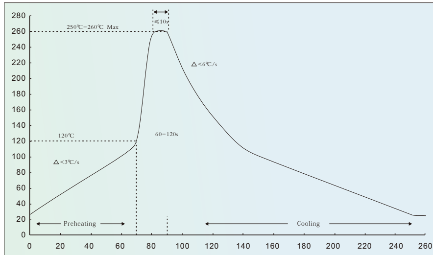
图二：波峰焊接温度曲线
