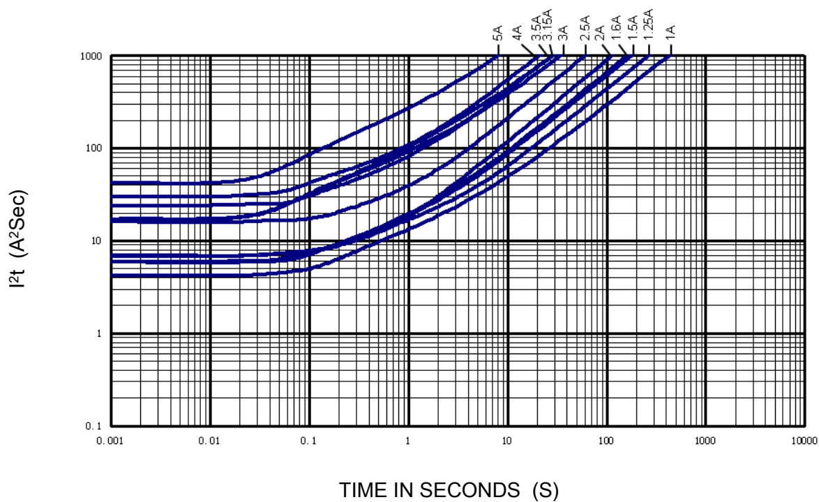
8-4 I^2t -t 圖/CHARACTERISTICS DIAGRAM( I^2t - t)
